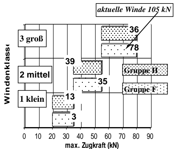
Abbildung: Anzahl bisher geprüfter Anbauwinden Gruppe H = Handhebel-/Zugleinenbedienung Gruppe F = Funkfernbedienbar Stand: Mai 2016
